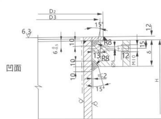
衬环凹凸密封面 NB/T 47022-2012(JB/T 4702)
