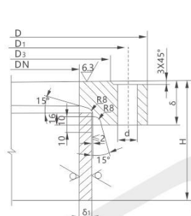
平密封面法兰
