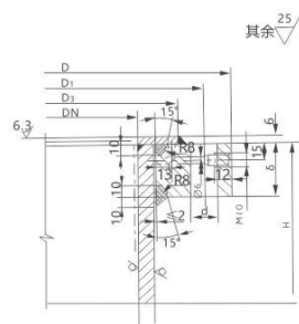
衬环平密封法兰 NB/T 47022-2012(JB/T 4702)
