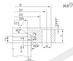
平密封面法兰
