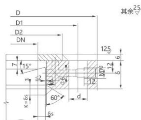
衬环平密封面 NB/T 47021-2012(JB/T 4701)
