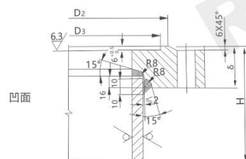
凹凸密封面法兰
