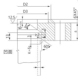
凹凸密封面法兰
