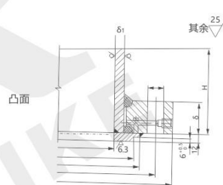
衬环平密封法兰 NB/T 47022-2012(JB/T 4702)
