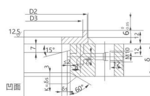
衬环凹凸密封面 NB/T 47021-2012(JB/T 4701)
